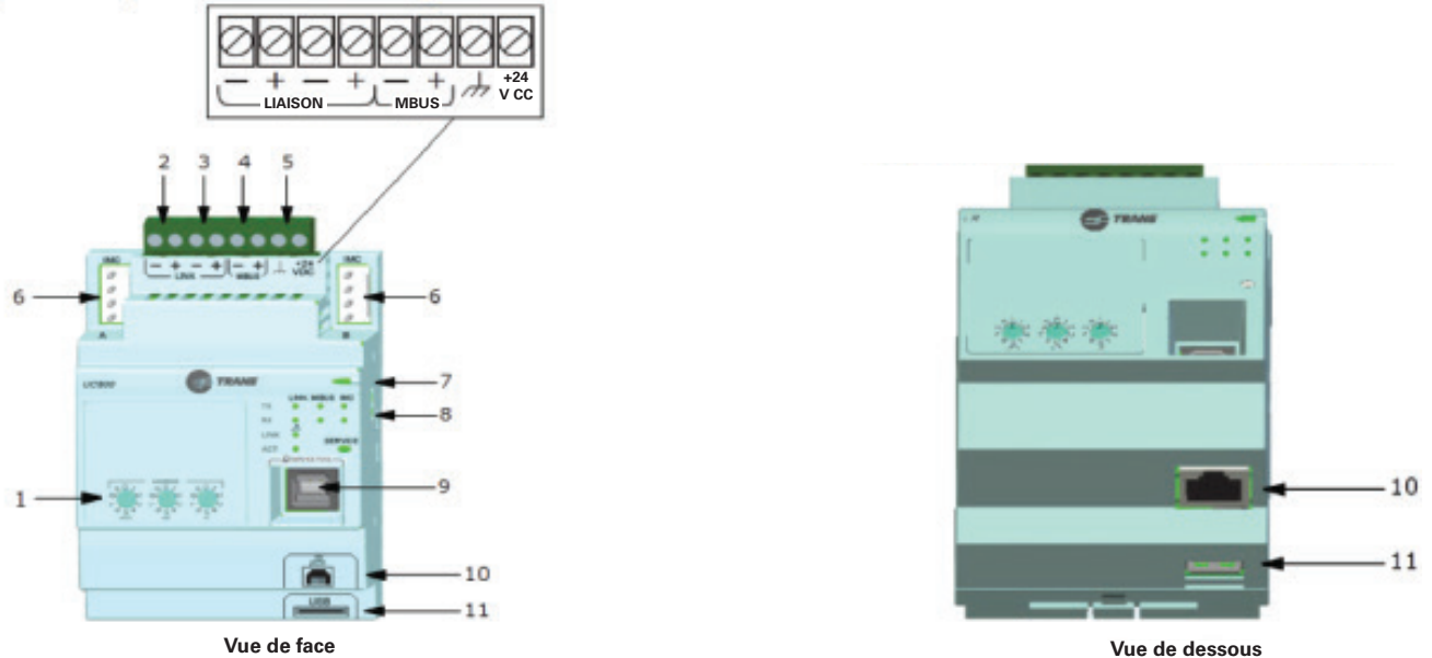
Figure 1 - Emplacements des câbles et ports de connexion du contrôleur UC800
