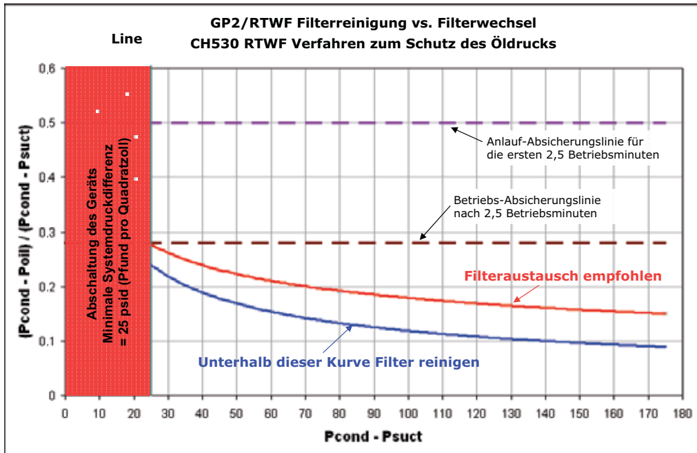
Abbildung 10 – Diagramm zum Ölfilterwechsel für RTWF
