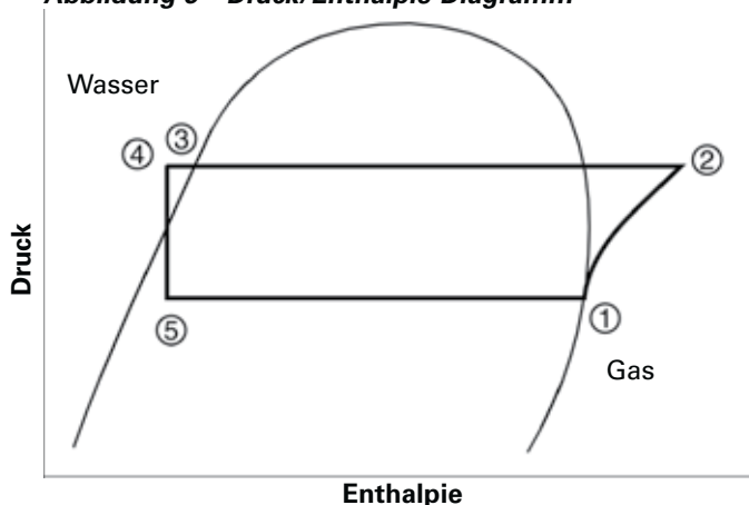
Abbildung 6 – Druck/Enthalpie-Diagramm
