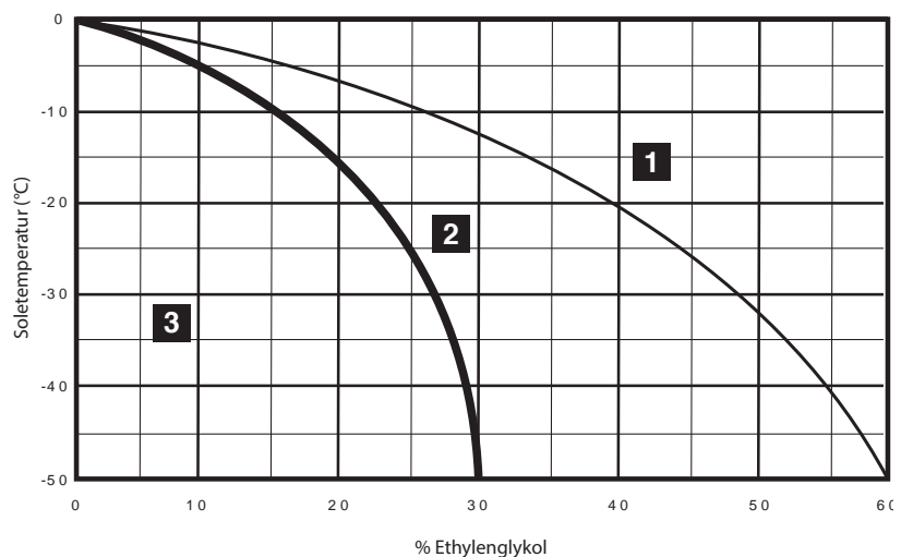
Abbildung 4 – Gefrierpunkt im Verhältnis zum prozentualen Ethylenglykol-Anteil
